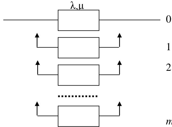
Рис. 4.6. Структурная схема резервированной системы
