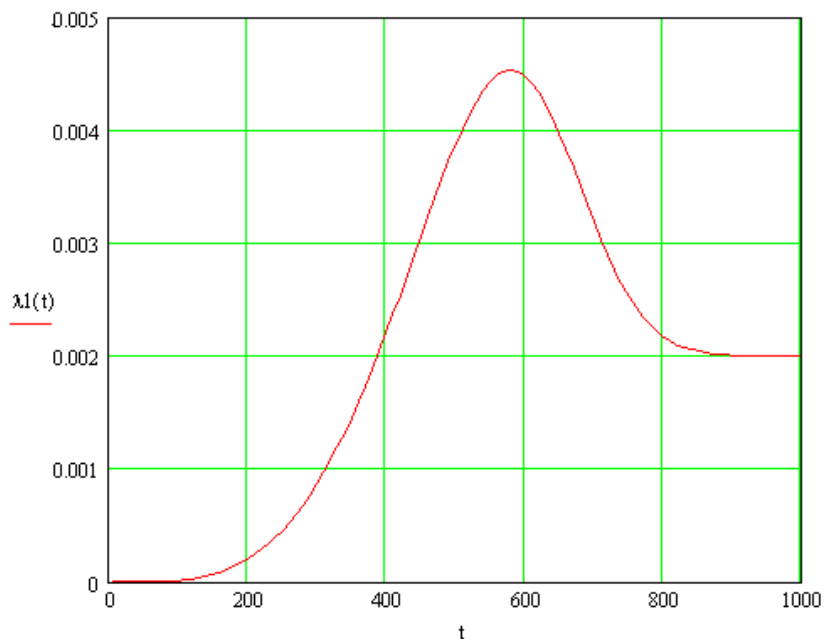
Рис. 3.6. Интенсивность отказа системы
