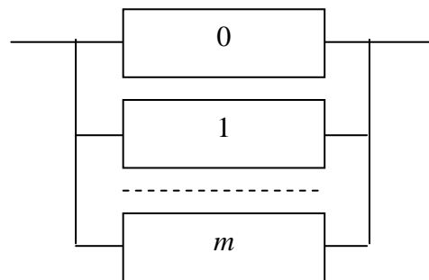
Рис. 3.2. Резервированная система с постоянно включенным резервом
