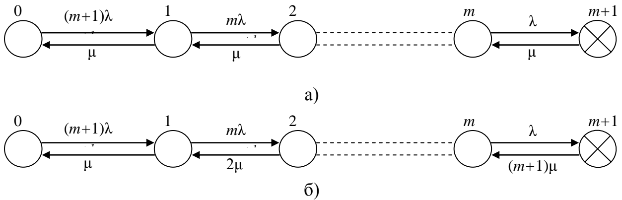
Рис. 4.5. Графы состояний резервированной системы: одна бригада обслуживания (а), (m+1) бригада обслуживания (б)
