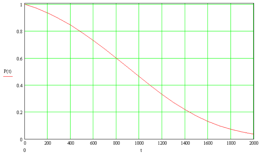
Рис. 2.8. Вероятность безотказной работы системы в течение t = 2000 часов
