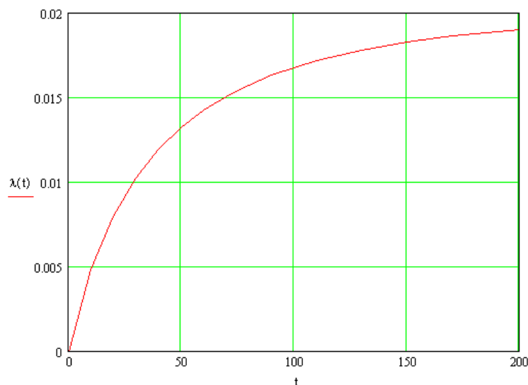
Рис. 3.8. Зависимость интенсивности отказов мажоритарной системы от времени
