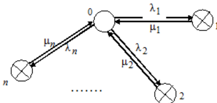
Рис. 4.1. Граф состояний системы с основным соединением элементов
