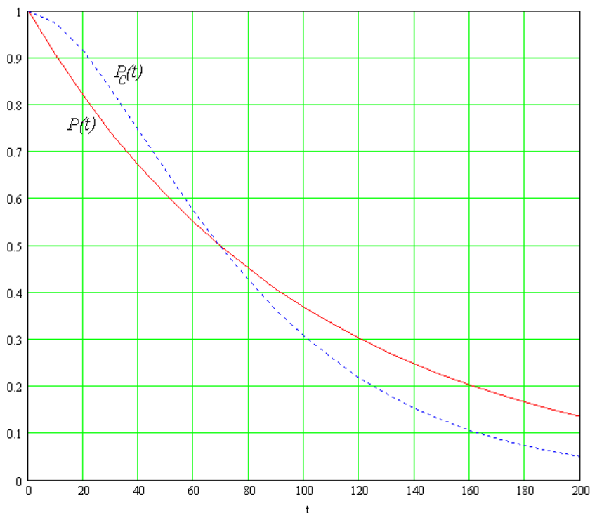
Рис. 3.7. Зависимости вероятности безотказной работы системы от времени
