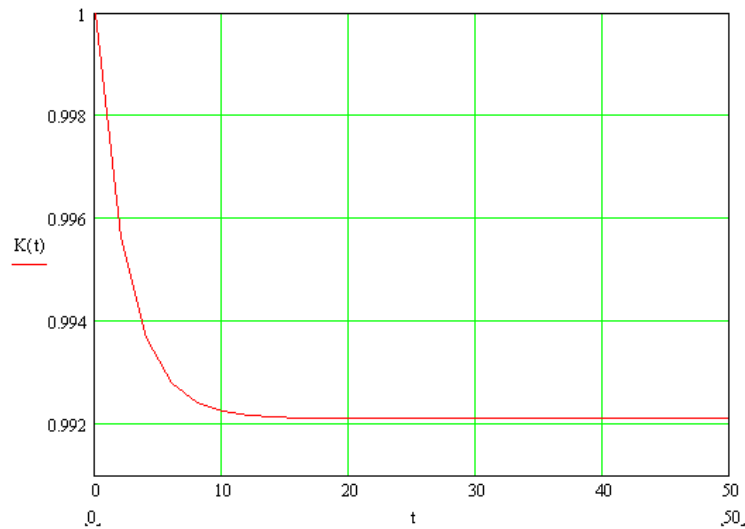
Рис. 4.2. Функция готовности системы
