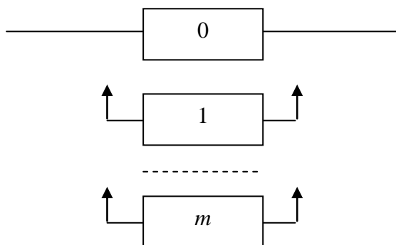
Рис. 3.9. Резервированная система с резервом замещением
