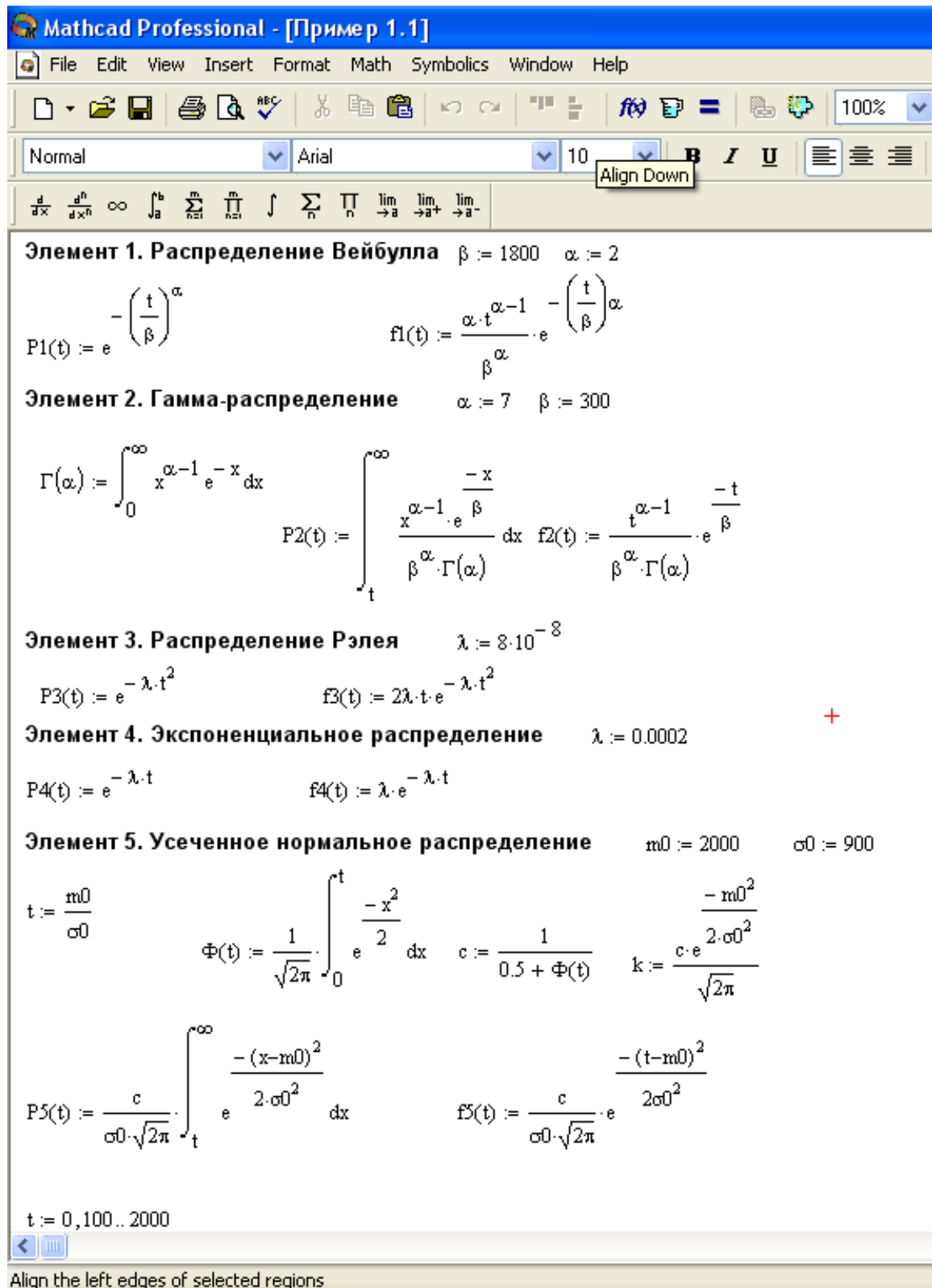
Рис. 2.6. Вычисление вероятности безотказной работы и плотности распределения
