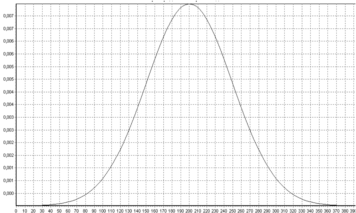
Рис. 2.3. Плотность нормального распределения
