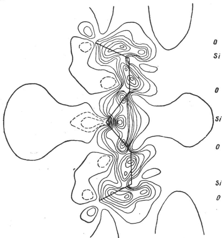
Рис. 19. Распределение электронной плотности (ДЭП) вдоль макромолекулярной цепочки связи Si-O-Si для кварца ( \alpha – \text{SiO}_2 )
