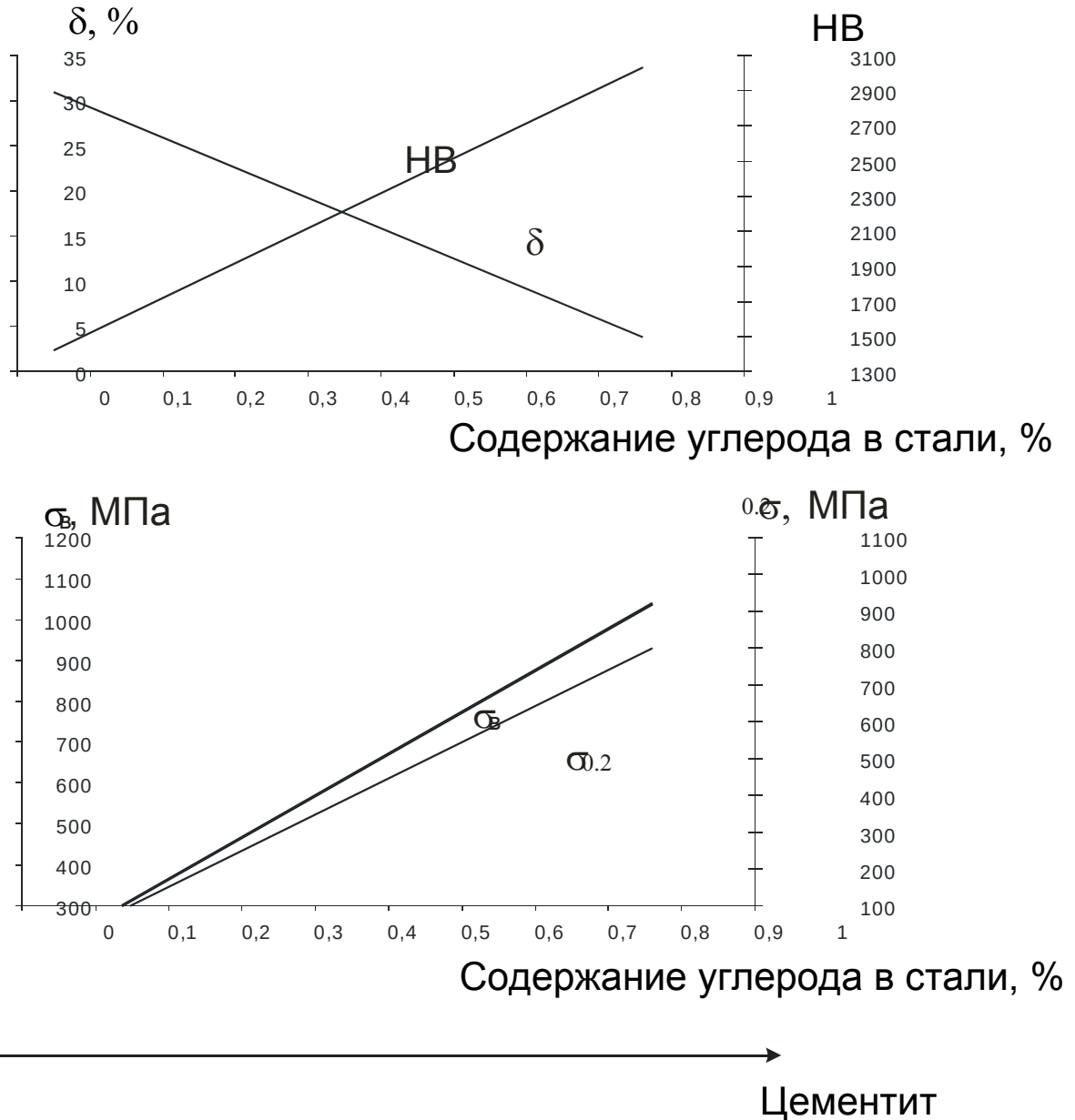
Рис. 72. Зависимость некоторых свойств углеродных сталей от содержания углерода
