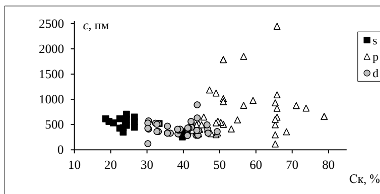
Рис. 71 (б). Зависимость периода идентичности b от C_K материалов на основе гомоядерных химических соединений
