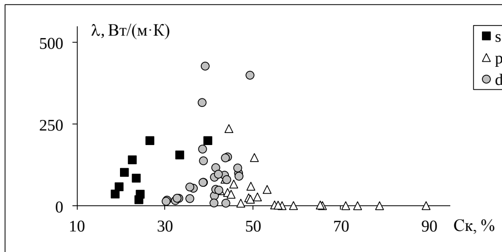
Рис. 69. Зависимость теплопроводности \lambda от C_k материалов на основе гомоядерных химических соединений
