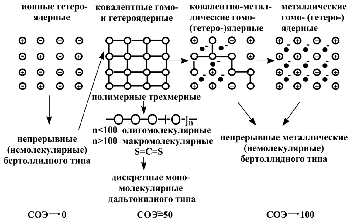
Рис. 47. Схематическое изображение различных типов химических структур, веществ и материалов на их основе
