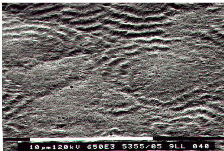
Рис. 58. Сферолитическая морфология полиэтилена низкой плотности, полученного из 40 мас. %-ого раствора в декалине ( \times 6500 )
