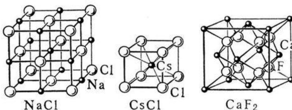
Рис. 50. Строение некоторых ионных кристаллов
