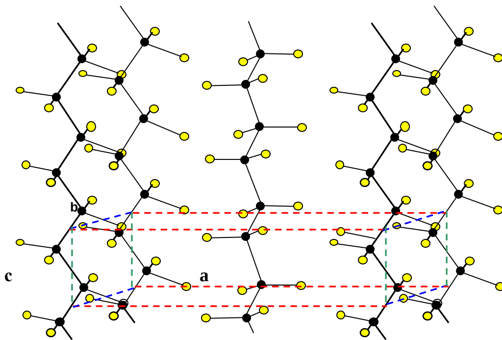
Рис. 53. Орторомбическая структура кристалла полиэтилена
