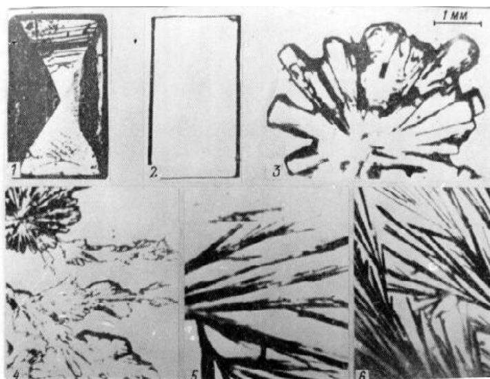
Рис. 61. Характерные формы кристаллов, образующихся при испарении водных растворов системы \text{Na}_5\text{P}_3\text{O}_{10} - (\text{NH}_4)_5\text{P}_3\text{O}_{10} - \text{H}_2\text{O} (0,2 мол. 20^\circ\text{C} ):
