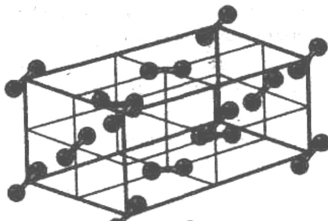
Рис. 51. Молекулярная структура кристалла иода
