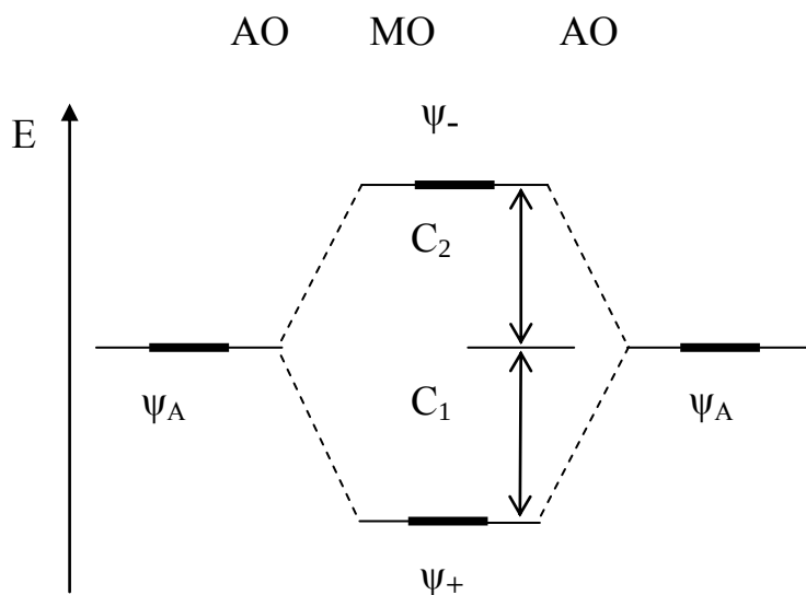
Рис. 27 (б). Энергетическая диаграмма атомных и молекулярных уровней тонкой структуры гомоядерного водородоподобного соединения
