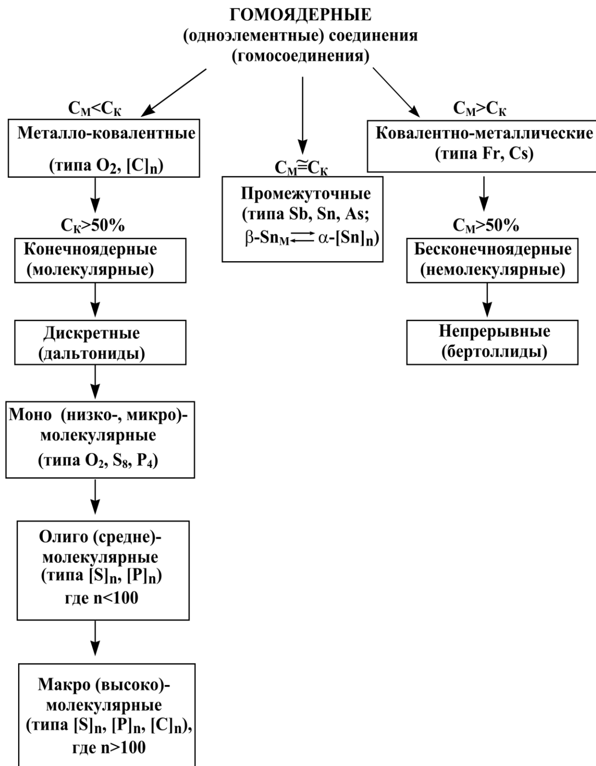
Рис. 45. Классификация гомоядерных (одноэлементных) соединений, веществ и материалов по преобладающему типу химической связи и другим производным характеристикам, где n – число ядер (атомных остовов) в молекулярных соединениях, М – металличность
