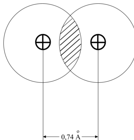
Рис. 15. Перекрывание электронных оболочек при образовании молекулы \text{H}_2
