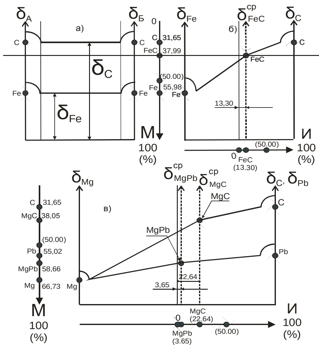
Рис. 36. Величины электронной плотности ( \delta ) и характер ее распределения в межъядерном пространстве для связей: а) Fe-Fe и C-C; б) Fe-C; в) Mg-C и Mg-Pb, где М – металличность, И – ионность
