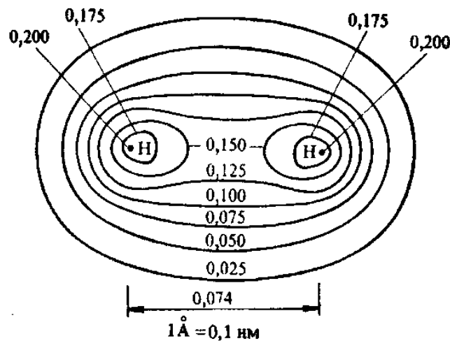
Рис. 21. Карта распределения электронной плотности молекулы водорода
