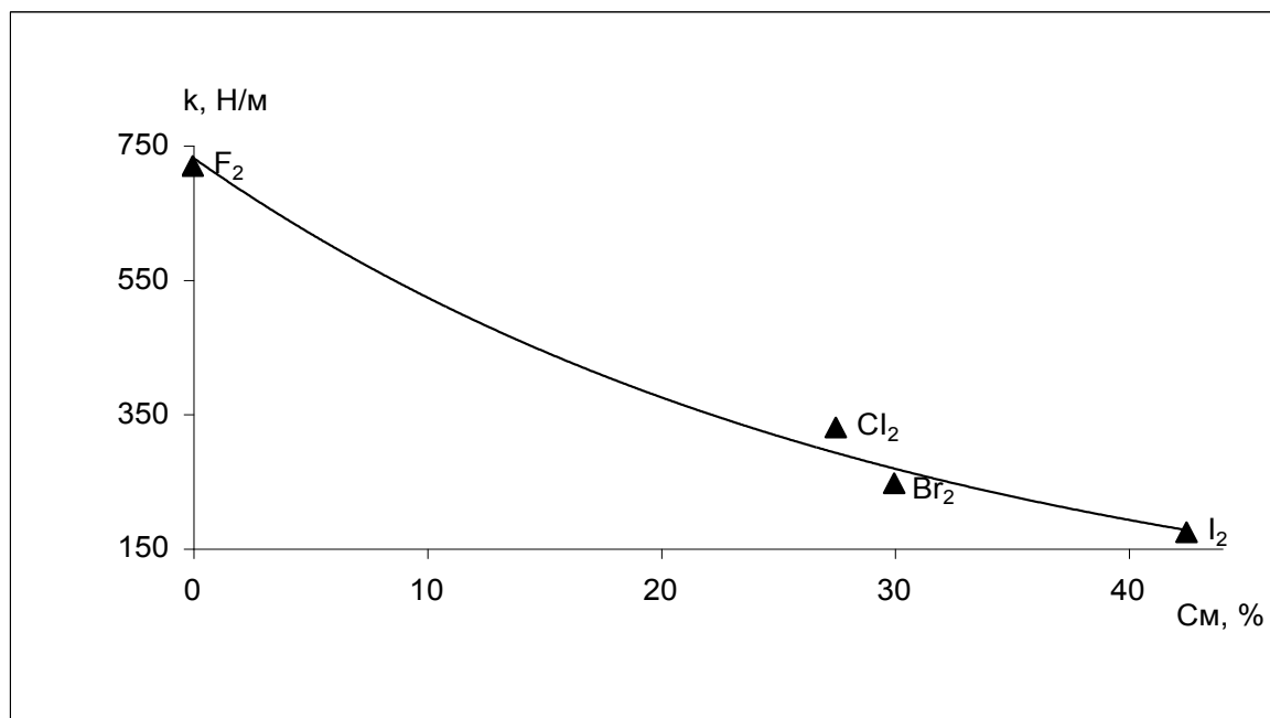
Рис. 36. Силовая константа химической связи ( k ) в галогенах как функция ее степени металличности ( C_M )
