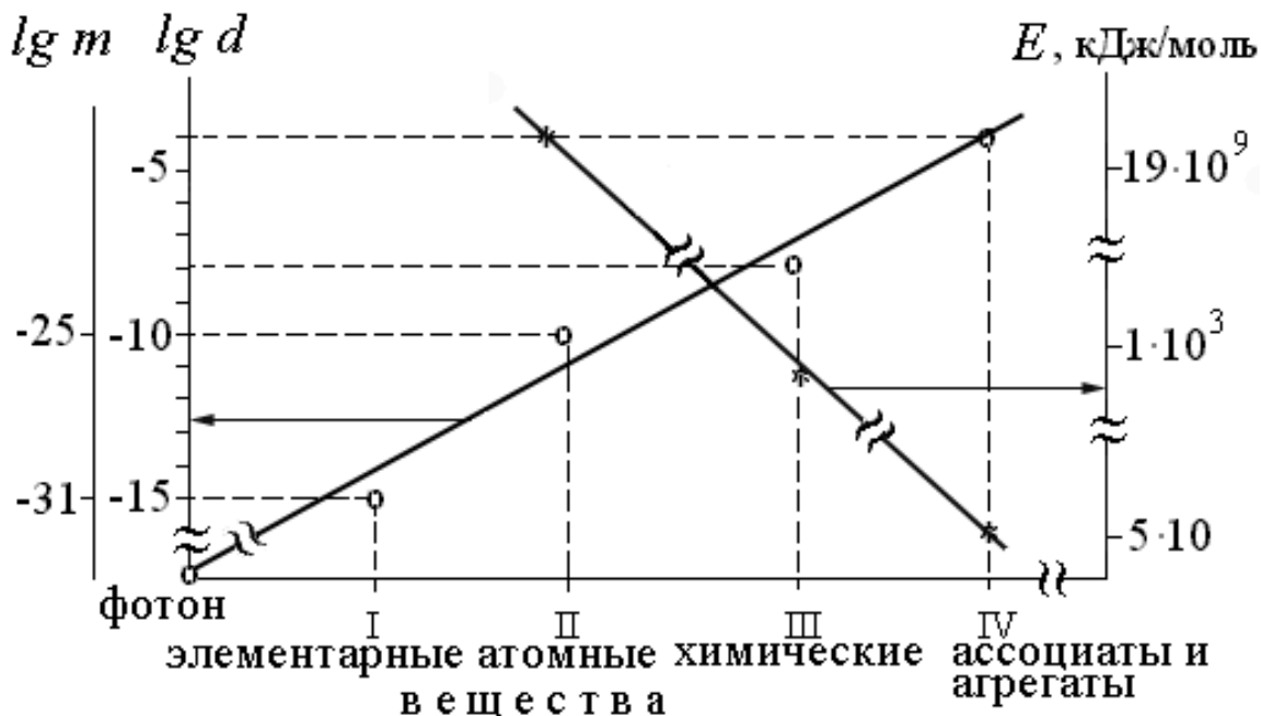
Рис. 4. Размерно-массовые и энергетические характеристики внутриструктурного взаимодействия частиц различных уровней организации вещества (единицы измерения массы m – кг, диаметра частиц d – м)
