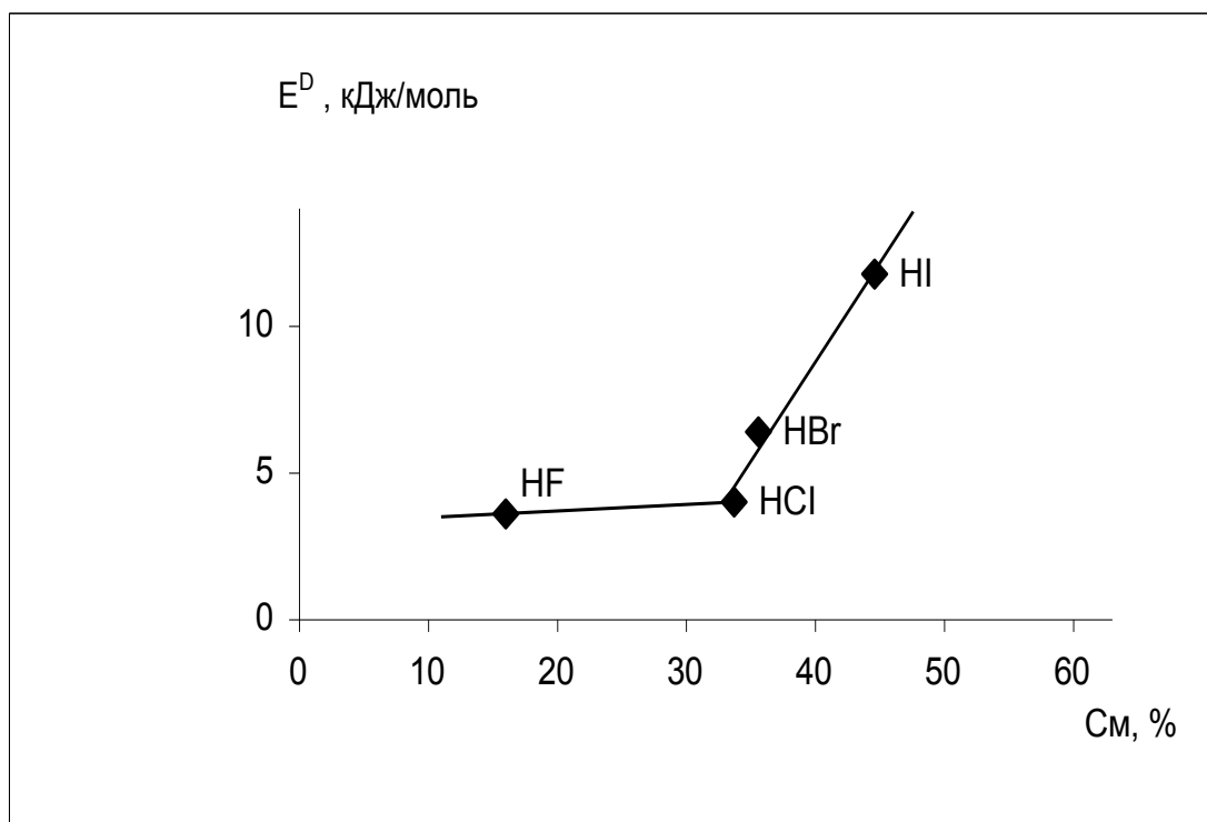
Рис. 38. Влияние степени металличности ( C_M ) на дисперсионную компоненту ММВ E^D для галогеноводородов
