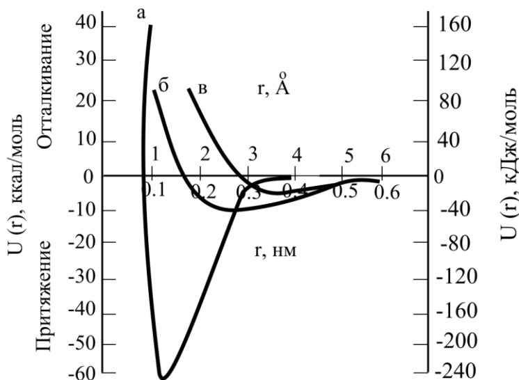
Рис. 20. Кривые потенциальной энергии межъядерных (химических) и межмолекулярных (физических) взаимодействий: а – ковалентная химическая связь; б – водородная связь; в – ван-дер-ваальсовая связь
