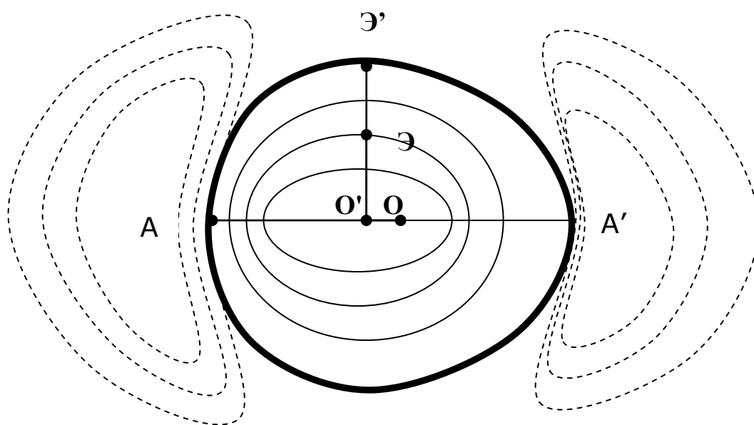
Рис. 28 ( a ). Диаграмма распределения электронной плотности в гетероядерном соединении
