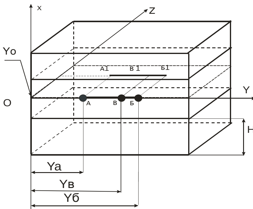
Рис. 34. Система координат для двух ядер в тонкой структуре материала в соответствии с программой Gaussian 94 W
