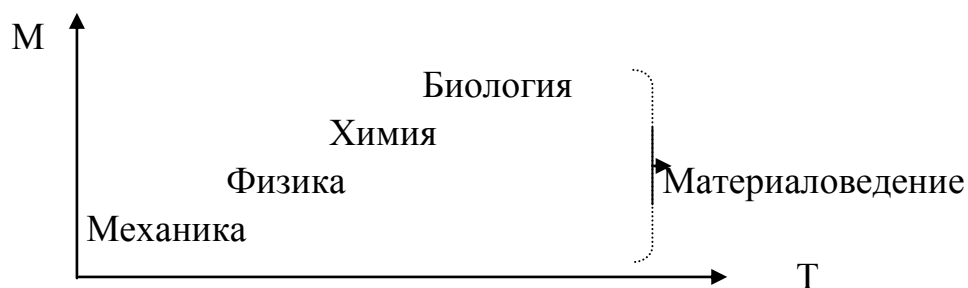
Рис. 8. Иерархия основных естественных наук, по Кекуле, дополненная материаловедением, как производной от них комплексной (симбиозной) дисциплиной
