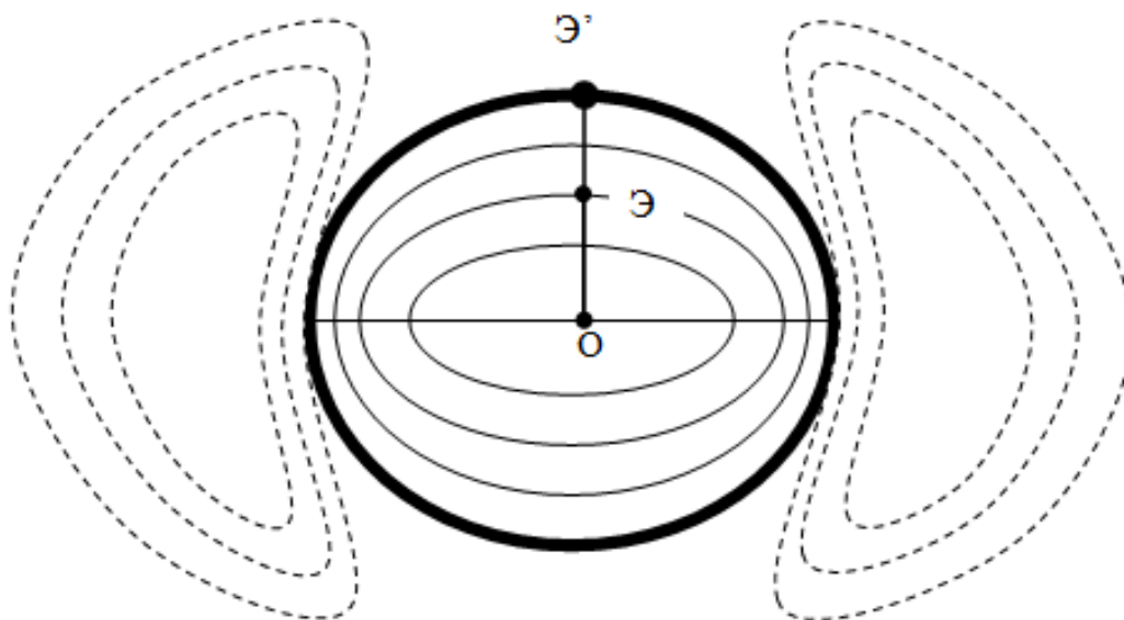
Рис. 27 (а). Разностная зарядовая плотность в молекуле H_2
