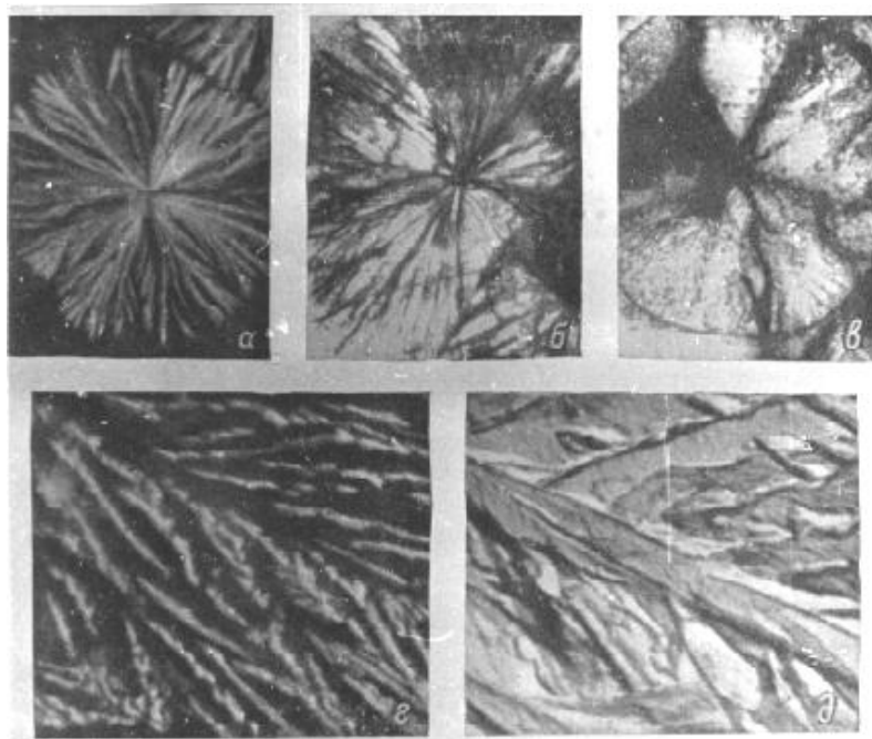
Рис. 59. Примеры надмолекулярных структур в углеродных и неуглеродных полимерных веществах: а – полипропилен, \times 400 ; б – дисиликат лития, \times 400 ; в – неорганическое стекло «анортит»; з – полипропилен, \times 1000 ; д – дисиликат лития, \times 700
