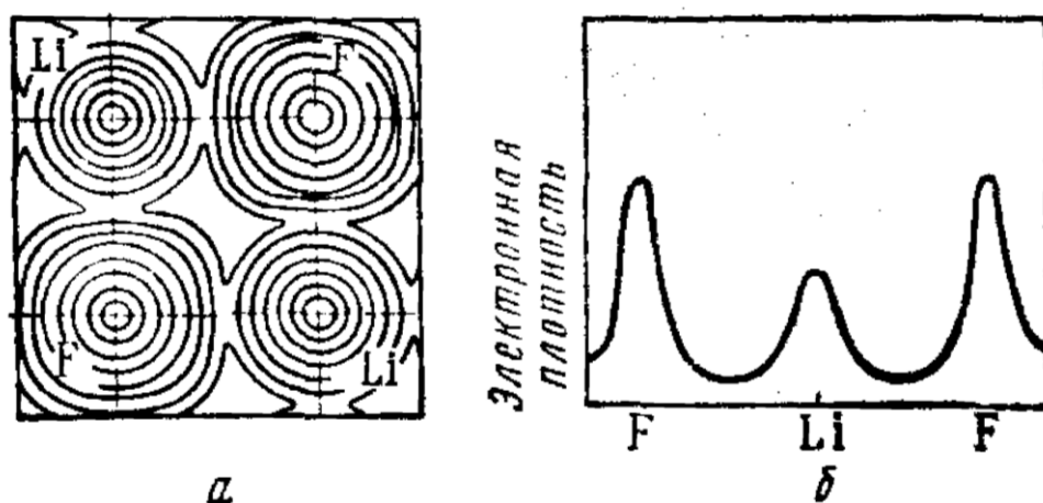
Рис. 24. Распределение электронной плотности между атомами в кристалле фторида лития: a – линии изоэлектронной плотности; б – зависимость электронной плотности от межатомных расстояний
