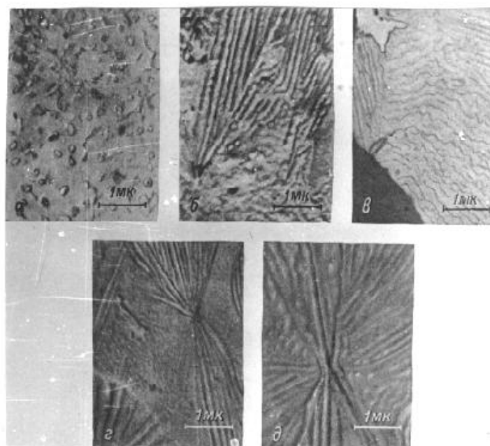
Рис. 60. Образование сферолитов при кристаллизации стекла состава анортита (состав, мас. %: \text{SiO}_2 – 43,2; \text{Al}_2\text{O}_3 – 36,7; \text{CaO} – 20,1): а – t = 980^\circ\text{C} , \tau = 4 ч; б, в – разные участки t = 980^\circ\text{C} , \tau = 4 ч 20 мин; г – 980^\circ\text{C} , \tau = 4 ч 30 мин; д – 980^\circ\text{C} , \tau = 5 ч
