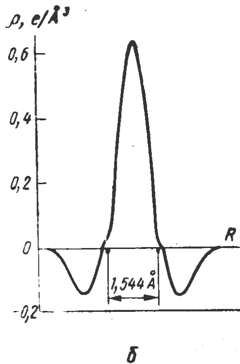
Рис. 18. Сечение ДЭП в кристалле кремния (а); избыточная плотность валентных электронов вдоль направления связи С-С в кристалле алмаза (б)
