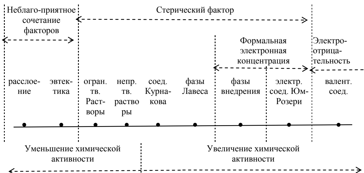
Рис. 54. Влияние металлохимических факторов на увеличение химического сродства по Я.А. Угаю
