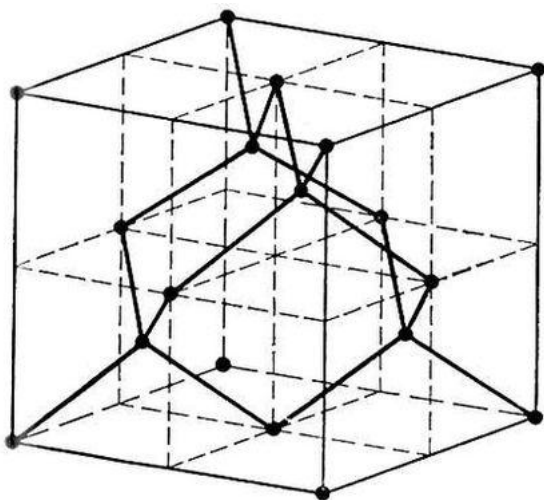
Рис. 49. Элементарная ячейка кристаллической решетки алмаза
