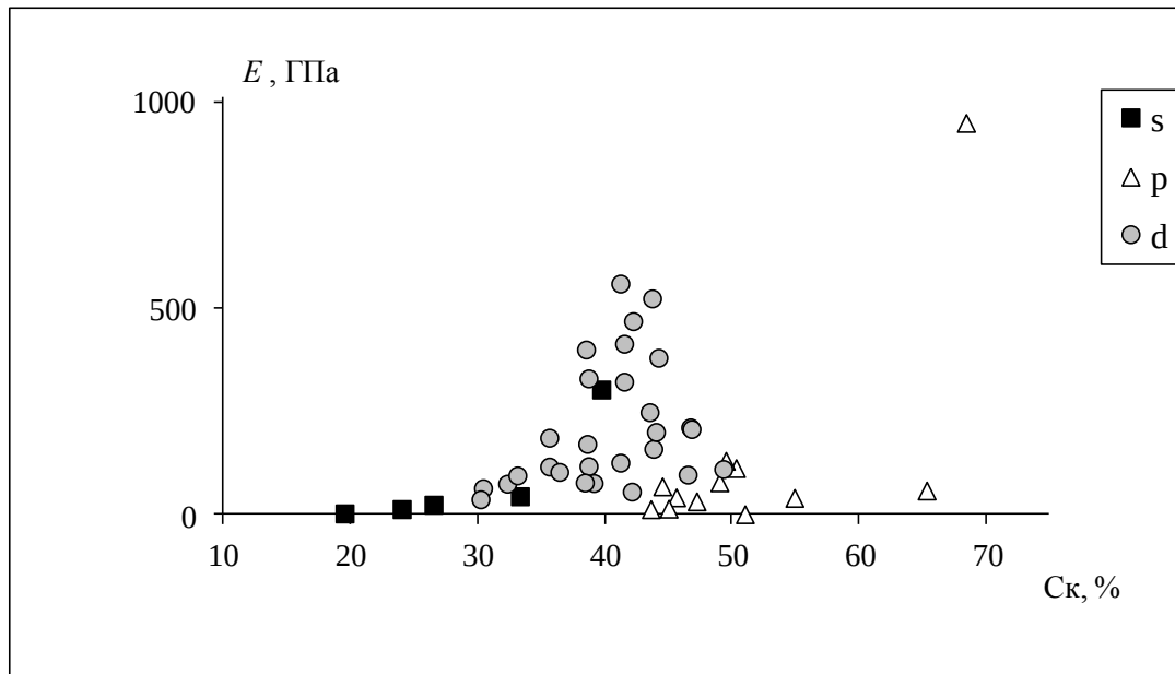
Рис. 62. Зависимость модуля упругости E от C_K материалов на основе гомоядерных химических соединений
