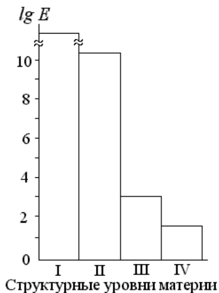
Рис. 5. Энергия внутривещного взаимодействия частиц и уровни организации вещественной материи (единицы измерения E – кДж/моль): I – ультрамикрорфизический, II – микрорфизический, III – химический, IV – «макрорфизический» – надмолекулярный
