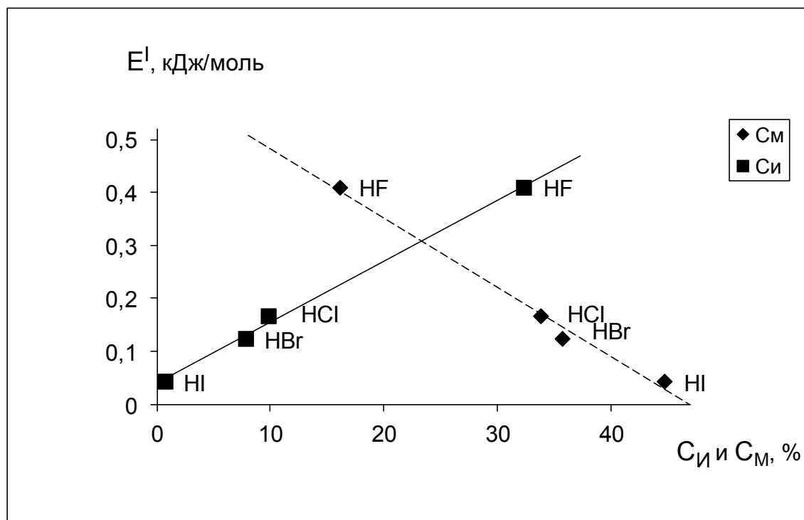
Рис. 40. Влияние степеней ионности C_{\text{И}} и металличности C_{\text{М}} на индукционную компоненту ММВ E^{\text{I}} для галогеноводородов
