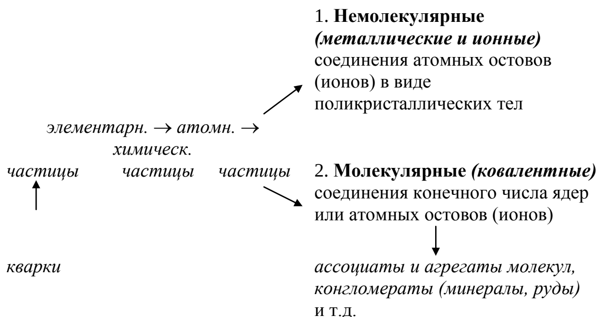
Рис. 3. Схема усложнения частиц вещественной материи Микромира
