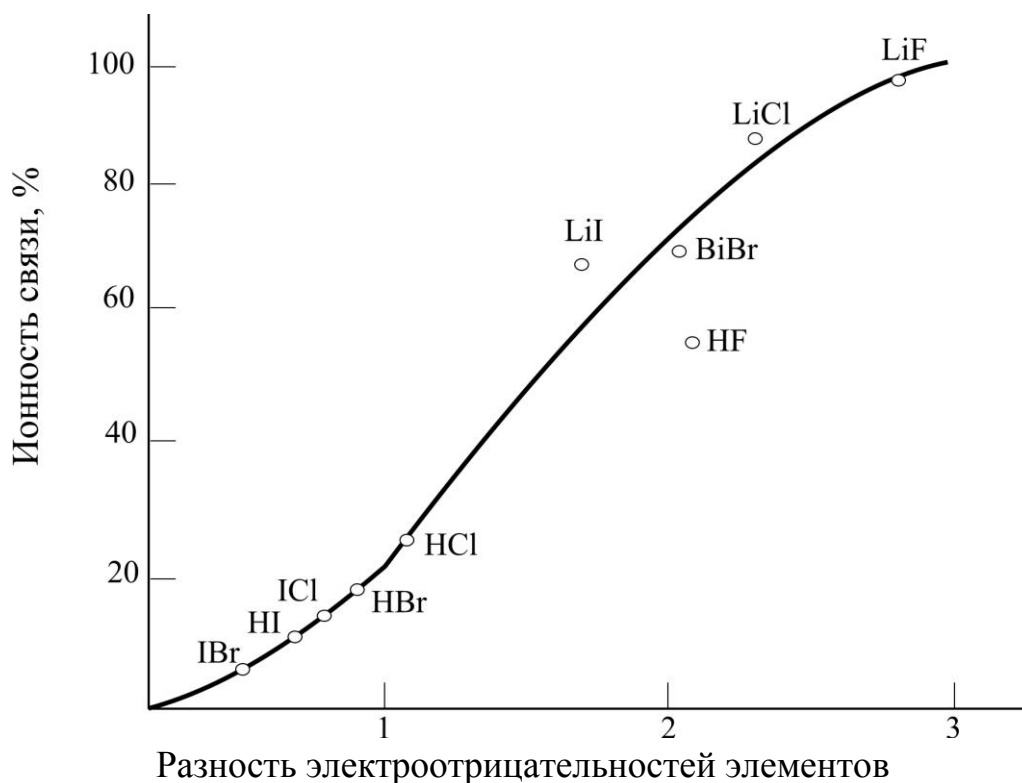
Рис. 31. Влияние разности электроотрицательностей элементов А и Б ( X_A - X_B ) в гетеросоединениях на степень ионности их связи
