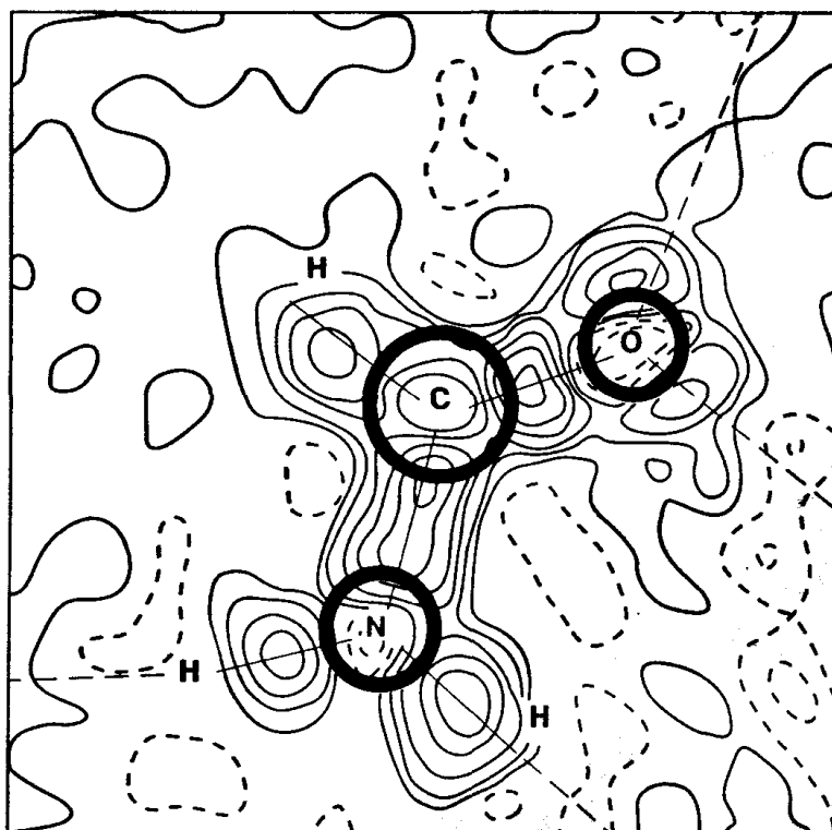
Рис. 17. Сечение деформационной электронной плотности, проходящее через среднюю плоскость молекулы в кристалле формамида \text{NH}_2\text{--CHO}
