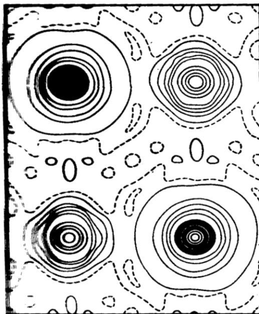
Рис. 25. Диаграмма электронной плотности в межъядерном пространстве NaCl
