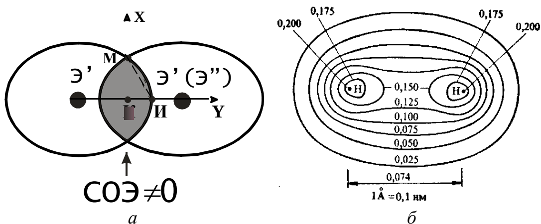
Рис. 29. Плоскостное изображение взаимосвязи ковалентной точка (K), вдоль оси X – металлической (M) и вдоль оси Y – ионной (II) составляющих (компонент) химической связи атомных остовов (ядер) гомо- ( Э' – Э'' ) и гетероядерных ( Э' – Э' ) структур (а) и карта электронной плотности гомоядерной молекулы H_2 (б)
