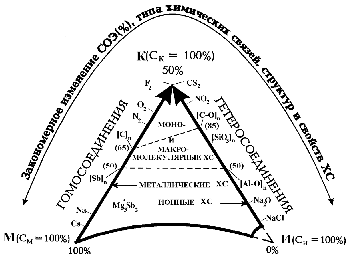
Рис. 42. «Химический треугольник» единства и различия химических связей и соединений (ХС) как основа для их систематизации
