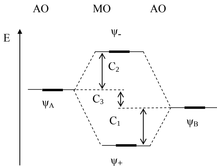
Рис. 28 (б). Энергетическая диаграмма атомных и молекулярных уровней тонкой структуры гетероядерного соединения
