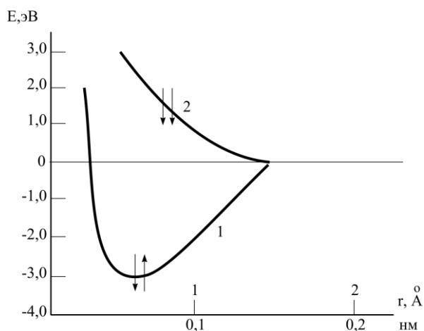
Рис. 14. Изменение потенциальной энергии системы двух атомов водорода: 1 – атомы водорода с разными спинами; 2 – атомы водорода с одинаково направленными спинами
