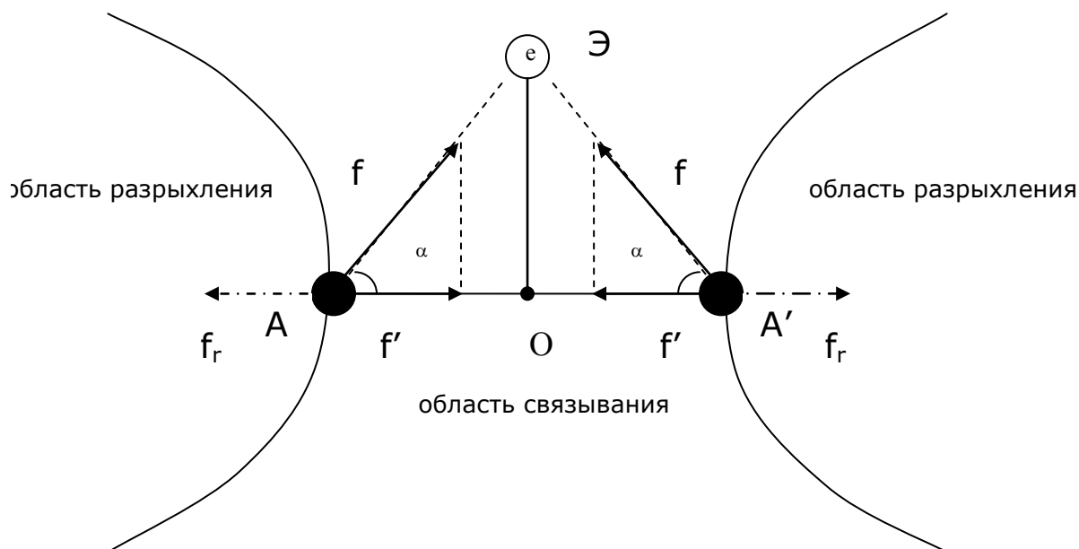
Рис. 26. Взаимодействие (связь) ядер А и электроном в молекуле H_2
