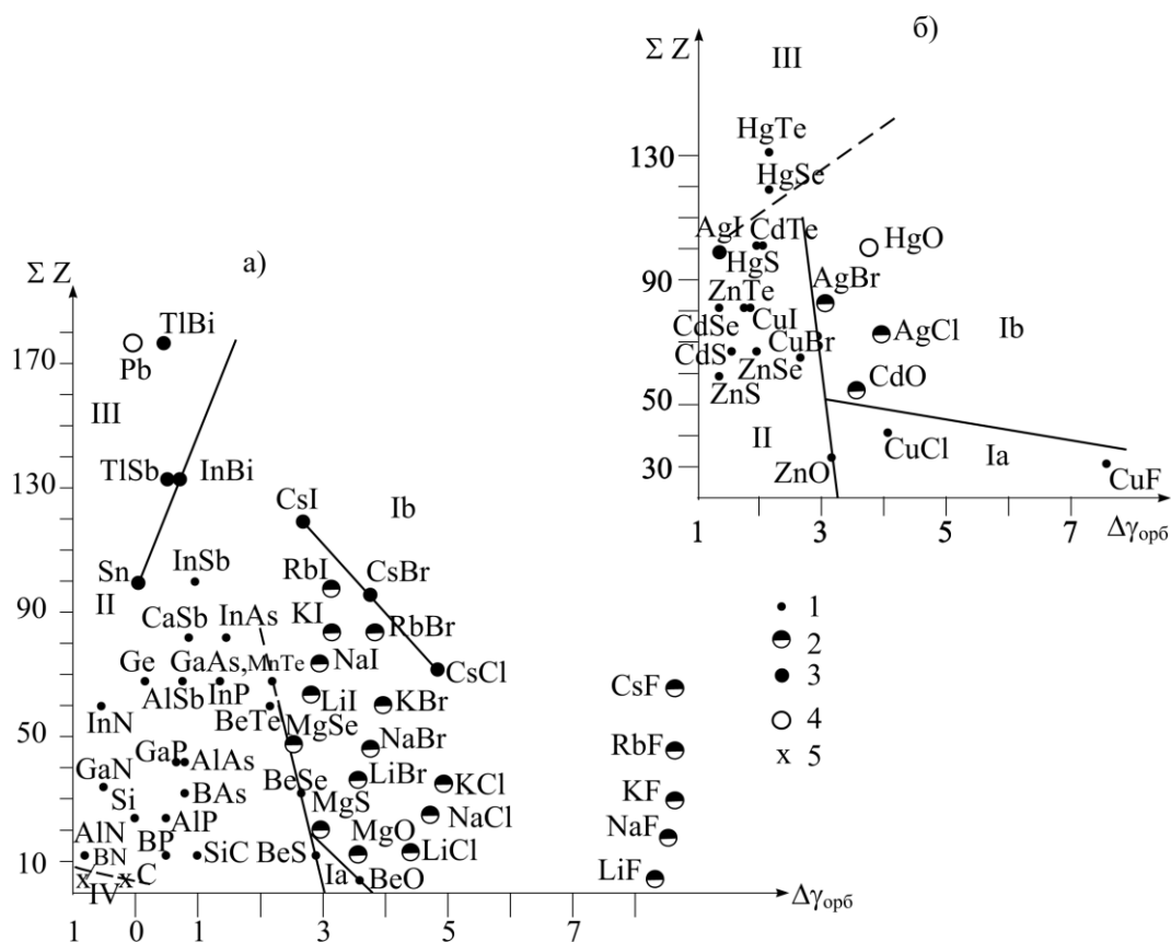
Рис. 33. Тип химической связи и структура гетероядерных веществ A^N B^{8-N} как функция суммарного атомного номера \Sigma Z и разности силовых характеристик \Delta \varphi_{\text{орб}} , определяющих степень металличности и степень ионности связи, переход от ковалентных кристаллов (II) к ионным (I), металлическим (III), молекулярным (IV). В поле ионных кристаллов выделены поля кристаллов со структурой типа BeO-CuCl (КЧ = 4), NaCl-AgCl (КЧ = 6), CsCl (КЧ = 8), обозначенные как Ia, Ib и Ib соответственно: а – вещества, в которых А – s- и p-элементам; б – вещества, в которых А = d-элементам; 1 – структуры с КЧ = 4; 2 – с КЧ = 6; 4 – с иной структурой; 5 – структуры типа графита
