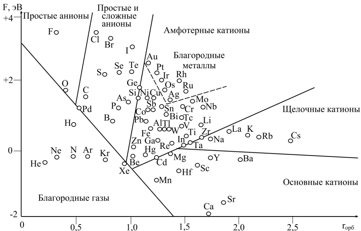
Рис. 32. Связь между F и r_{орб} элементов
