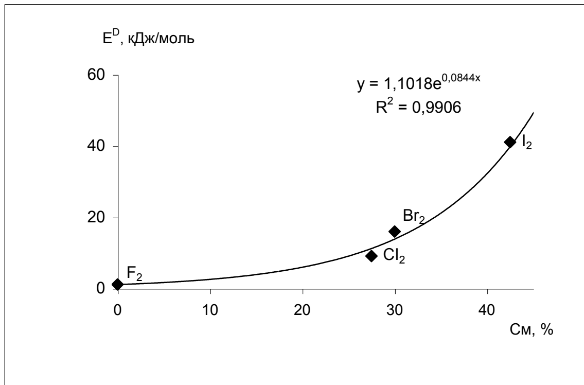
Рис. 37. Влияние степени металличности ( C_M ) химической связи на энергию ВДВ взаимодействия E^D для галогенов
