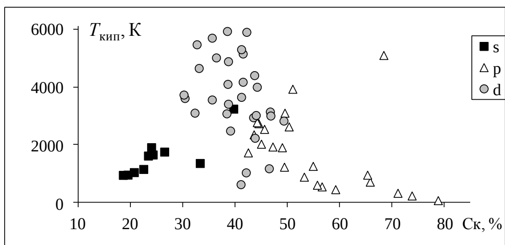
Рис. 67. Зависимость температуры кипения T_{\text{кип}} от C_{\text{к}} материалов на основе гомоядерных химических соединений
