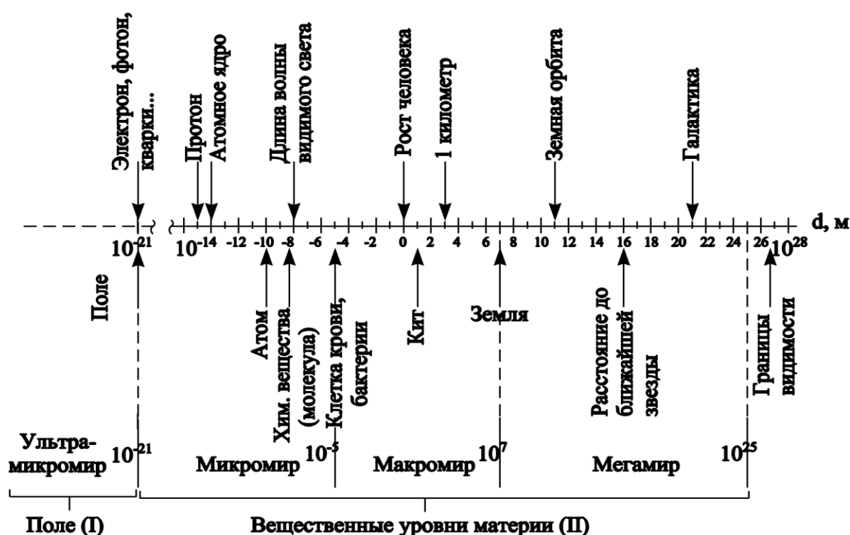
Рис. 7. Общая классификация материальных объектов Мироздания по их размеру ( d ) к началу XXI в. ( d измеряется в метрах (м)), в рамках единой парадигмы многоуровневой организации материи и мироздания
