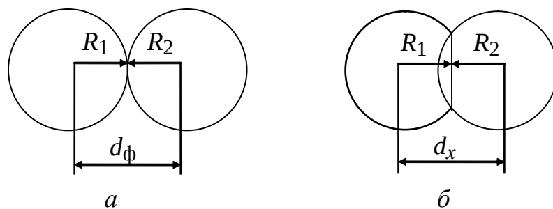
Рис. 13. Упрощенная модель физического ван-дер-ваальсового взаимодействия атомов (а) и механизма образования между ними химической связи в процессе физико-химического их превращения в процессе перекрывания электронных оболочек в биядерное химическое соединение – химическое вещество (б):
