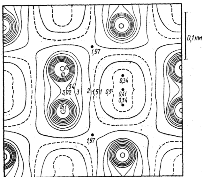
Рис. 22. Диаграмма электронной плотности между ядрами алмаза
