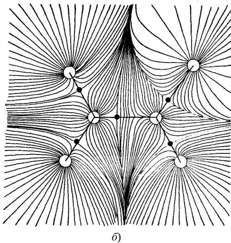
Рис. 16. Распределение электронной плотности в молекуле \text{CH}_2 = \text{CHF} : a – замкнутые изолинии соответствуют уровням функции \rho(r) ; б – градиентные траектории. На обоих рисунках дополнительно показаны линии связи, седловые точки (крупные черные точки) и поверхности нулевого потока
