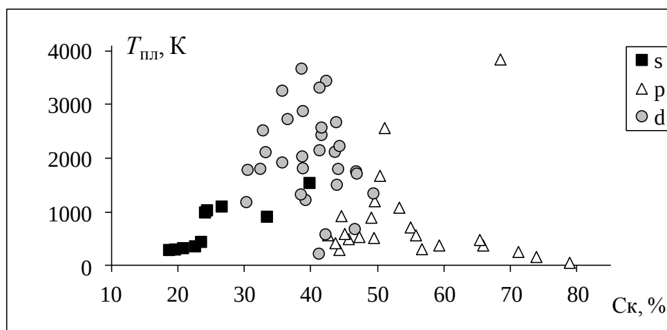
Рис. 66. Зависимость температуры плавления T_{\text{пл}} от C_{\text{к}} материалов на основе гомоядерных химических соединений
