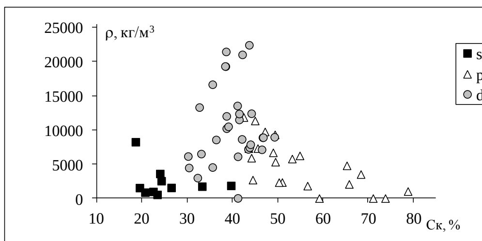
Рис. 68. Зависимость плотности \rho от C_{\text{к}} материалов на основе гомоядерных химических соединений
