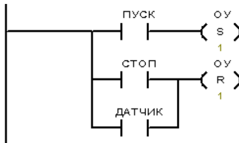
Рис. 1.11. Листинг программы
