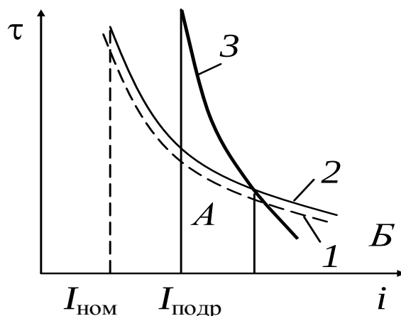
Рис. 8.1. Времятоковая характеристика
