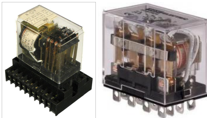
Рис. 12.5. Промежуточные реле различного исполнения
