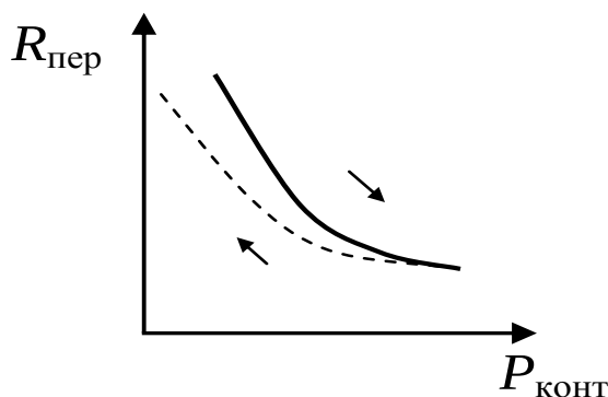
Рис. 4.1. Зависимость переходного сопротивления стягивания контакта от контактного нажатия
