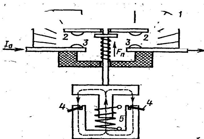
Рис.13.1. Прямоходовой контактор
