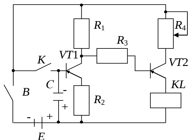
Рис. 12.7. Электрическая принципиальная схема реле времени
