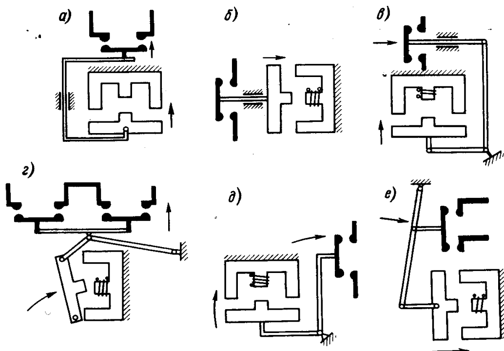
Рис. 13.2. Характерные кинематические схемы контакторов переменного тока нормального режима работы: а, б, в – прямоходовая схема; з, д, е – поворотная схема магнитной системы
