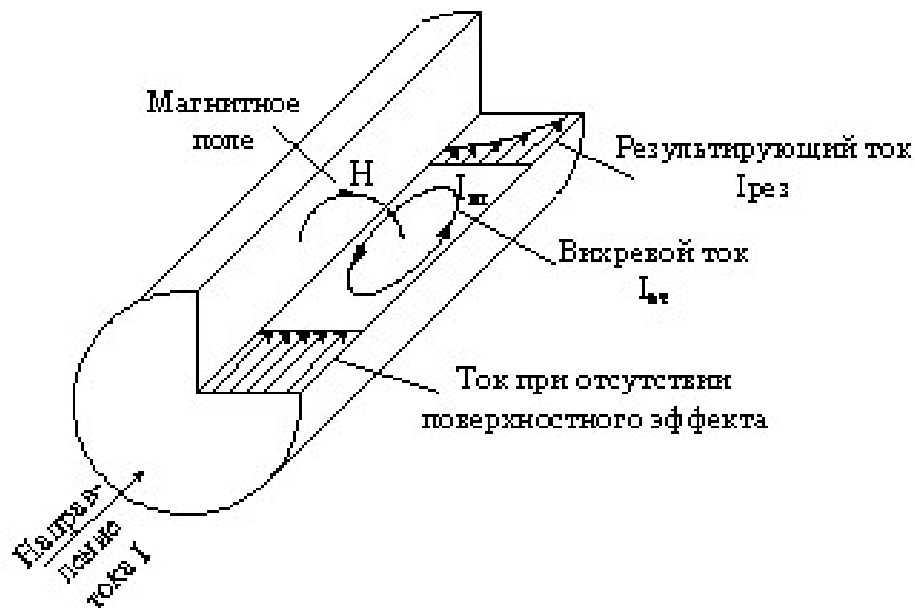
Рис. 2.5. Поверхностный эффект
