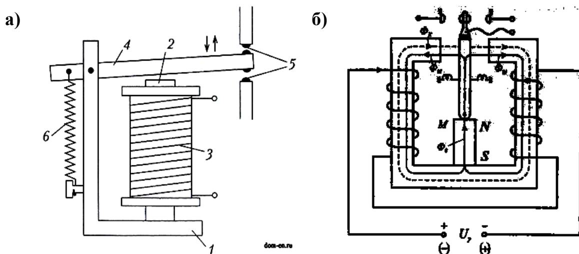
Рис. 12.2. Электромагнитные реле постоянного тока: а – нейтральное; б – поляризованное реле
